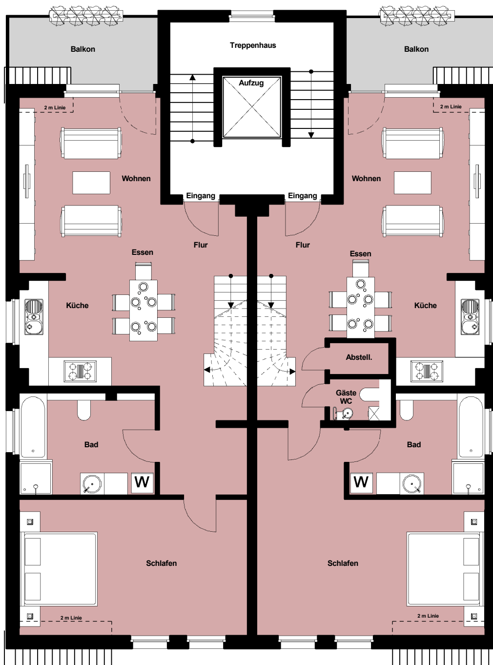
Dachgeschoss
